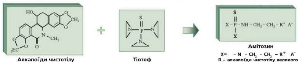
Схема одержання амітозину - першого представника нового наукового напрямку
